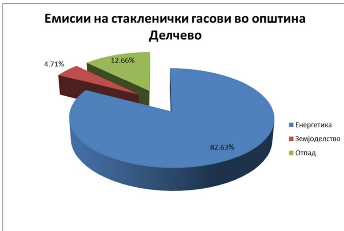
Слика 2. Процентуална застапеност на емисиите на стакленички гасови во Општина Делчево
